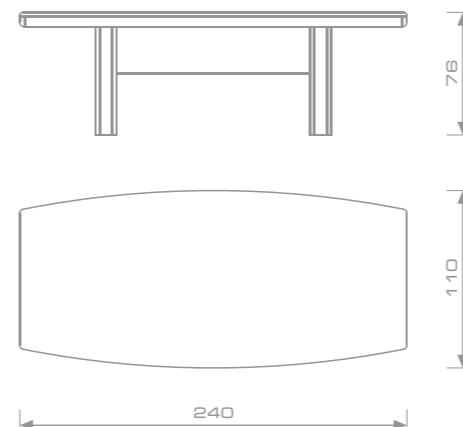
CONFERENCE TABLE. СТОЛ СОВЕЩАНИЙ RH 124 W240 D110 H76
