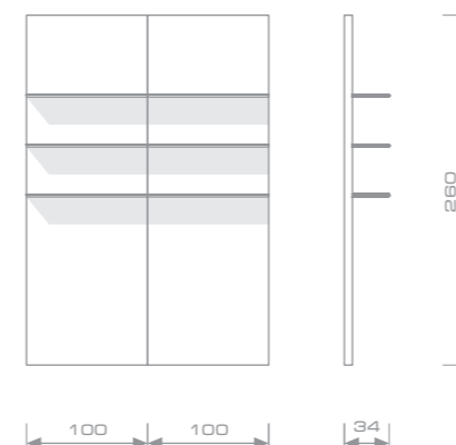
PANEL WITH THREE SPLIT SHELVES. СТЕНОВАЯ ПАНЕЛЬ С ТРЕМЯ ПОЛКАМИ MUX-P100A W100 D34 H260
