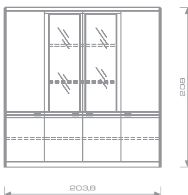
CABINET WITH GLASS AND WOODEN DOORS, COAT RACK. ШКАФ СО СТЕКЛЯНЫМИ И ДЕРЕВЯНЫМИ ДВЕРКАМИ, ВЕШАЛКА ДЛЯ ОДЕЖДЫ MUX 2020 W203,8 D47 H208
